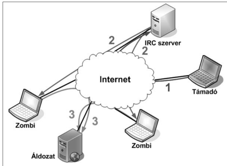
1. ábra Egy zombihálózat felépítése és a támadás folyamata
